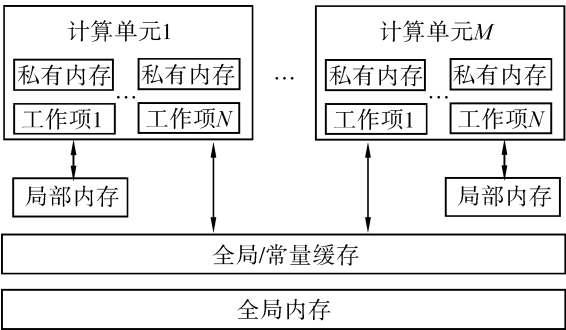
图 8 OpenCL 内存模型 Fig.8 OpenCL memory model
