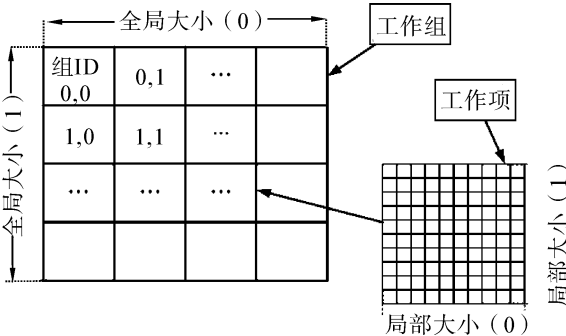
图 9 OpenCL 并行执行模型 Fig.9 OpenCL execution model
