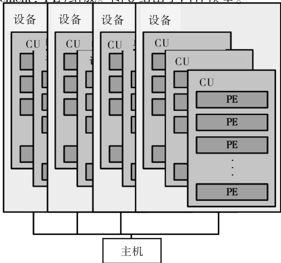
图 7 OpenCL 设备模型
